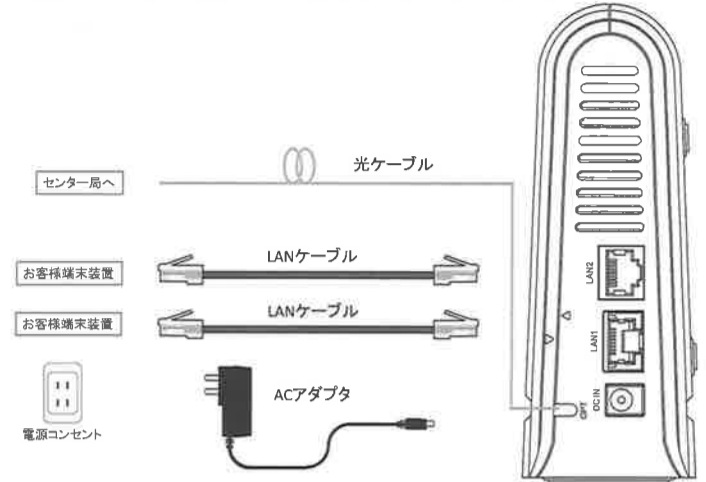
Fig.2 各種ケーブル接続構成図
