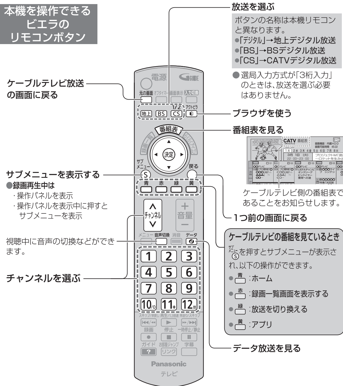
<ビエラのリモコン(例:TH-32A320)>
